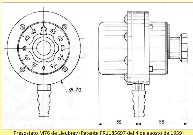
Presostato M76 de Lieubray (Patente FR1185697 del 4 de agosto de 1959)
