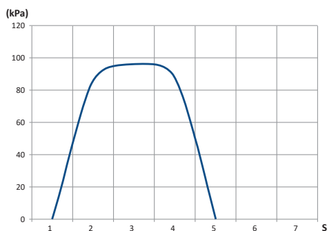
Gráfico de aumento de presión dentro de un pulsador de aire de 32 mm de diámetro (como el modelo 66ZM5 descrito en este catálogo)
